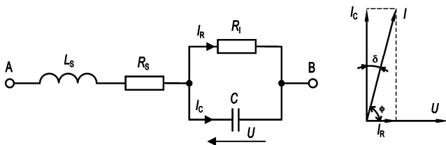
Rys. 2. Schemat zastępczy kondensatora o pojemności C , rezystancji upływności R_l , rezystancji szeregowej R_S i indukcyjności pasożytniczej L_S z wykresem wskazowym zależności fazowych między napięciem na kondensatorze U oraz jego prądem I_C ; I_R – prąd płynący przez rezystancję R_l
