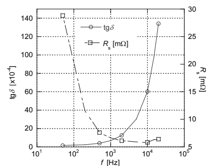
Rys. 4. Charakterystyki \text{tg}\delta i R_S w funkcji częstotliwości f pomierzone dla kondensatora typu MKSP-118 (7,5μF/425V) przy napięciu skutecznym polaryzacji 1V; pomiary wykonano mostkiem RLC GenRad 1689M Fig. 4. Characteristics of \text{tg}\delta and R_S vs. frequency f observed in a capacitor of type MKSP-118 (7,5μF/425V) at polarization of 1V rms voltage; measurements were taken with the RLC bridge GenRad 1689M
