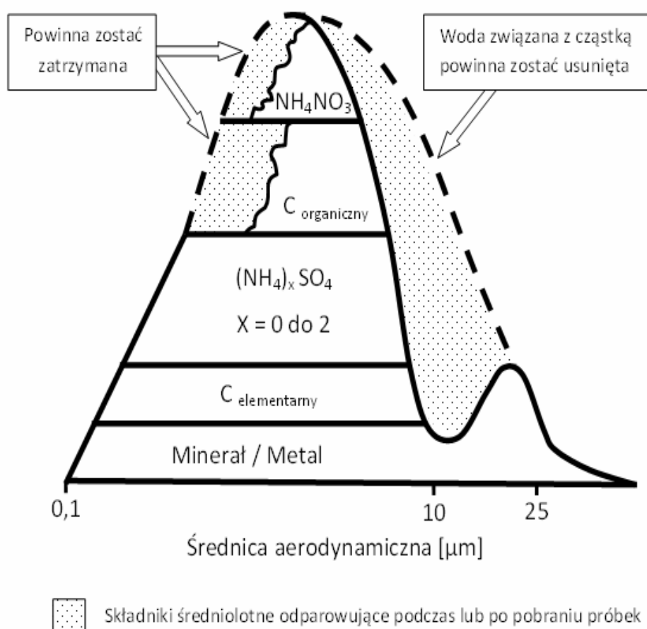
Rys. 2. Główne składniki średniolotne i nietlotne w PM_{2,5} [3]
