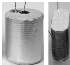
Rys. 5. Widok zwijek kondensatorów – walcowa (lewa) i spłaszczona (prawa) Fig. 5. Wound foils of capacitors – cylindrical (left) and flat (right)
