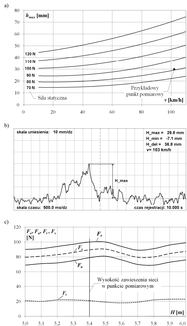
Rys. 7. Charakterystyki współpracy odbieraka z siecią: a) charakterystyki uniesienia przewodu jezdniego w zależności od siły statycznej odbieraka i prędkości jazdy; b) przebieg uniesienia przewodu dla wybranego odbieraka; c) charakterystyki statycznej siły nacisku przy obniżaniu F_o i unoszeniu F_u odbieraka, wartości siły średniej F_s , oraz podwójnej siły tarcia F_f – dla odbieraka z rys. b
