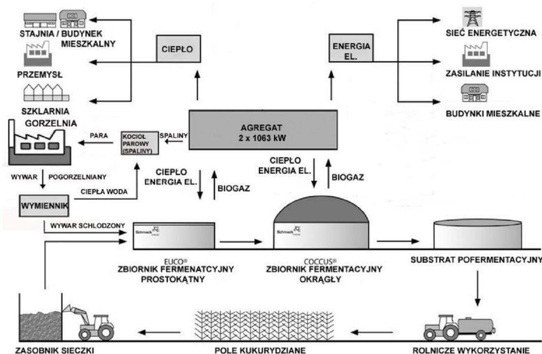
Rys. 3. Schemat instalacji wytwarzania i utylizacji biogazu w Gorzelnii Liszkowo [7] Fig. 3. Schema of biogas generation and utilisation system in Liszkowo Distillery [7]
