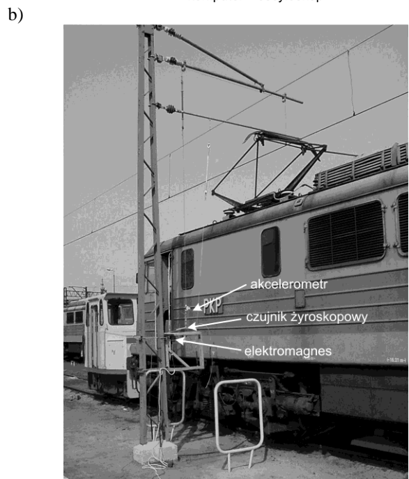
Rys. 12. Eksperymentalne terenowe stanowisko do badania stanu zawieszenia ślizgacza: a) szkic konstrukcyjny, b) widok stanowiska
