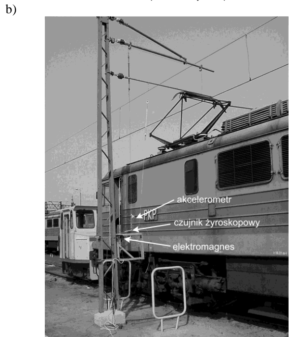
Rys. 12. Eksperymentalne terenowe stanowisko do badania stanu zawieszania ślizgacza: a) szkic konstrukcyjny, b) widok stanowiska
