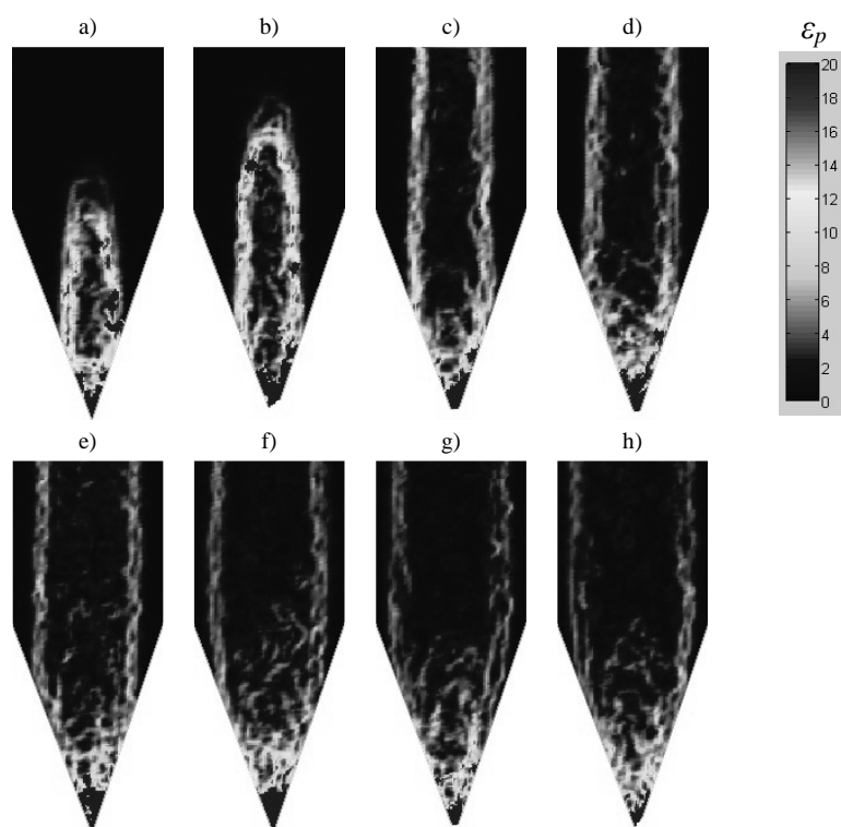
Rys. 7. Zmiana odkształceń postaciowych \varepsilon_p (nie sumowanych) w zagęszczonej piasku średnioziarnistym d_{50} = 0,8 mm w silosie ze ścianami bardzo szorstkimi i przepływem masowym:
