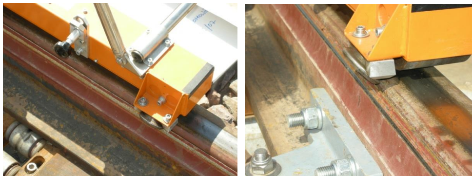
Fot. 7. Przejazd przez zwrotnicę prostą
