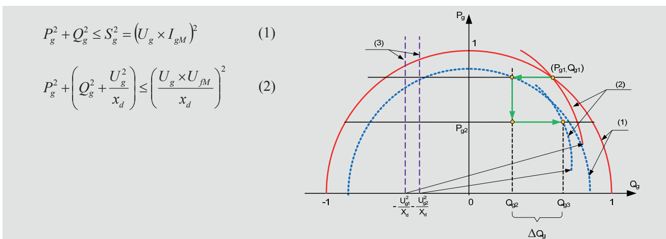
Rys. 5. Obszar dopuszczalnych stanów pracy generatora synchronicznego przy napięciu znamionowym (linie ciągłe) i przy napięciu mniejszym od znamionowego (linie przerywane). (1) – granica wynikająca z dopuszczalnej obciążalności prądowej stojana, (2) – granica wynikająca z dopuszczalnego napięcia (prądu) wzbudzenia, (3) – granica równowagi naturalnej (wynikająca z warunku zachowania stabilności). Dla uproszczenia na rysunku pokazano jedynie ograniczenia wynikające z dopuszczalnego prądu stojana i wirnika maszyny.
