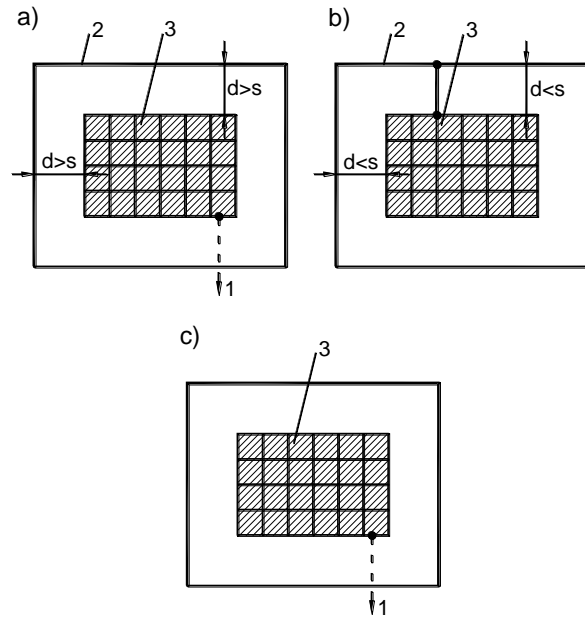
Rys. 3. Ochrona paneli PV zainstalowanych na dachach pochyłych przed bezpośrednim uderzeniem pioruna; 1 – przewód wyrównawczy bezpośredni do głównej szyny wyrównawczej potencjału, 2 – zwody poziome na kalenicy i krawędziach dachu, 3 – panel PV
