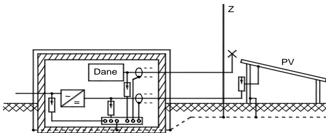
Rys. 8. Ochrona przeciwprzebieciowa systemów PV w elektrowni słonecznej, Z – zwód pionowy, X – układ do pomiaru warunków atmosferycznych, ~/= – falownik
