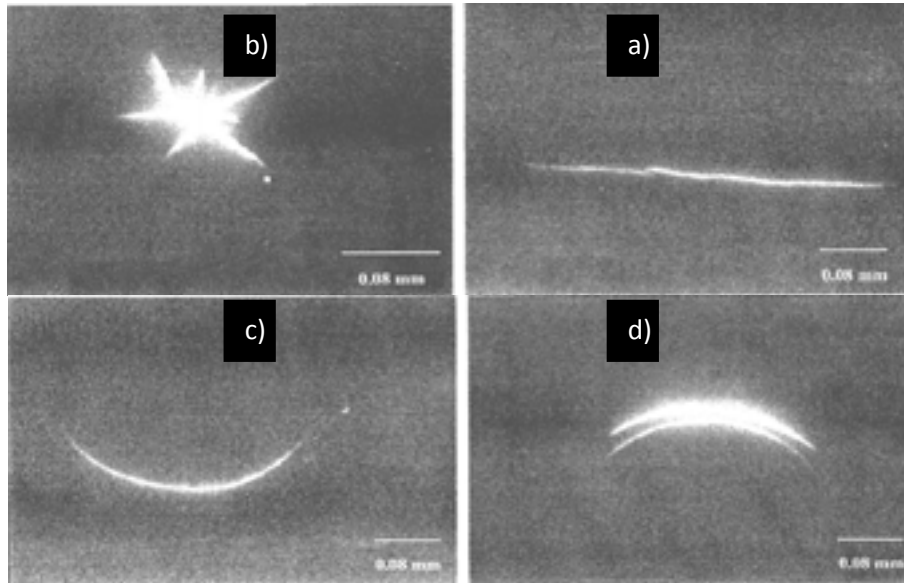
Rys. 1. Typowe wady spotykane na powierzchni kulek ceramicznych: a) pęknięcie gwiazdźdźiste, b) pęknięcie powstałe w wyniku procesu spiekania, c) pojedyncze pęknięcie koliste, d) wielokrotne pęknięcie koliste [L. 1]
