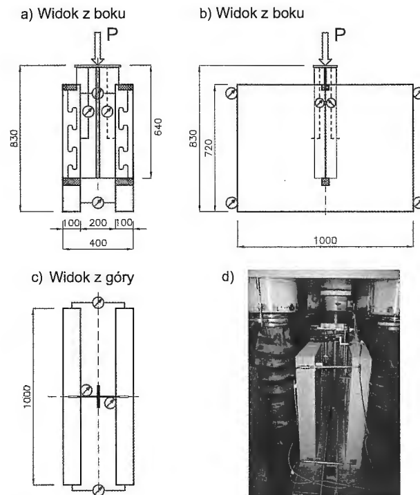
Rys. 5. Indukcyjne czujniki przemieszczeń zainstalowane na badanych elementach stalowo-betonowych: a), b), c) szkice rozmieszczenia czujników, d) element na stanowisku badawczym; widoczne dwa poziome i dwa pionowe czujniki
