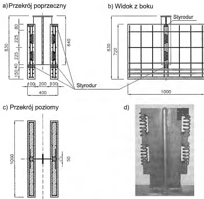
Rys. 3. Badane elementy stalowo-betonowe: a), b), c) szkice konstrukcji, d) widok średnika stalowego ze zbrojeniem uwzględniającym przed betonowaniem
