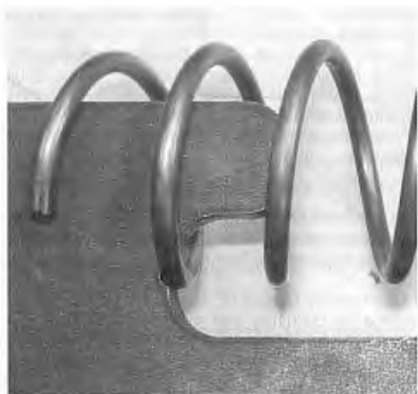
Rys. 4. Montaż zbrojenia uzwajającego na średnikach stalowych
