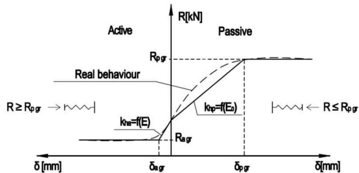
Fig. 1. Bilinear soil interaction dependence on the wall displacement. Rys. 1. Zależność reakcji gruntu od przemieszczeń obudowy wykopu
