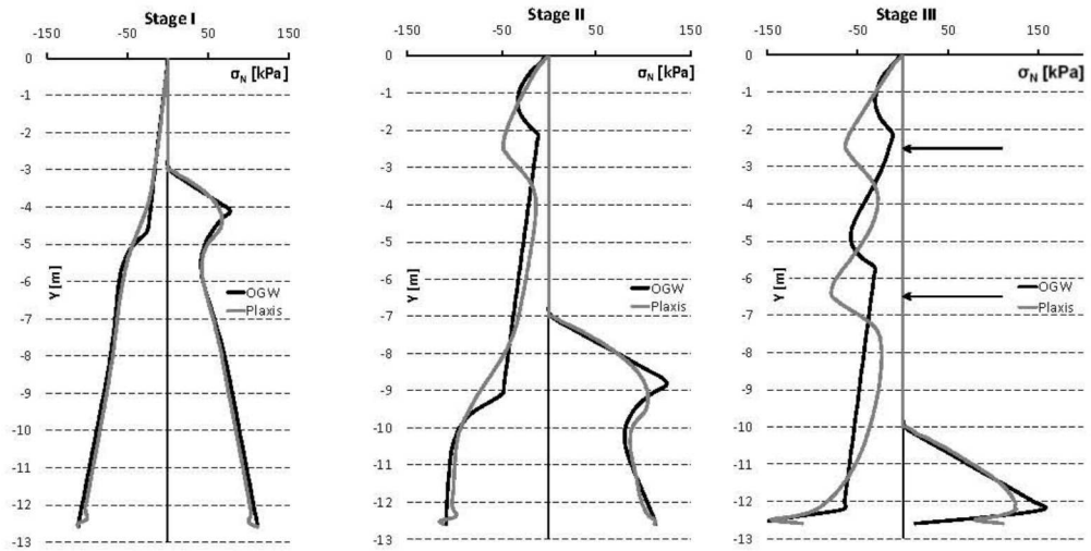
Fig. 11. Soil pressure acting on the sheet pile wall with struts. Rys. 11. Rozkłady parcia gruntu działającego na rozpiętą ściankę szczelną
