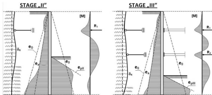
Fig. 2. The interaction between soil and wall modelled by elasto-plastic springs (OGW program). Rys. 2. Współpraca gruntu z obudową wykopu, wymodelowana za pomocą więzi sprężysto-plastycznych (program OGW)
