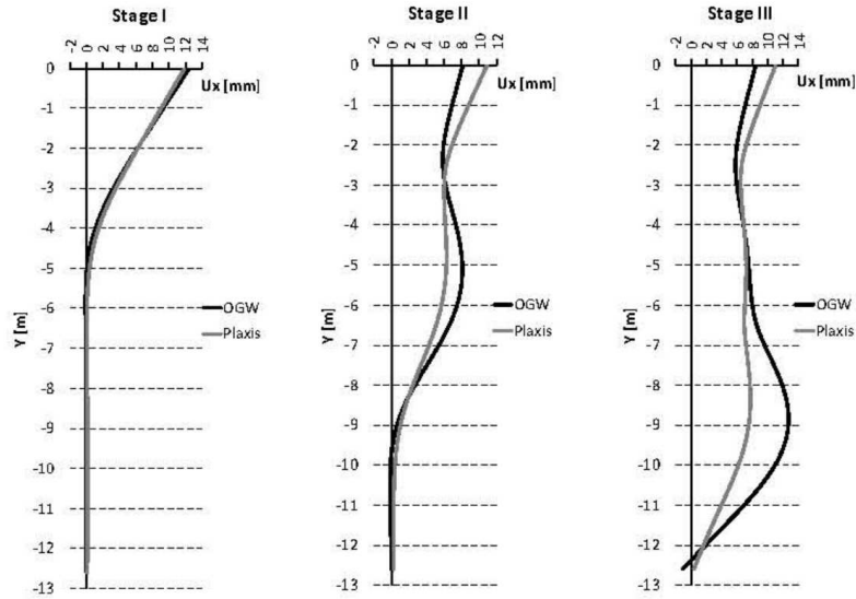
Fig. 10. Horizontal displacements of the sheet pile wall with struts. Rys. 10. Przemieszczenia poziome rozpiętej ścianki szczelnej
