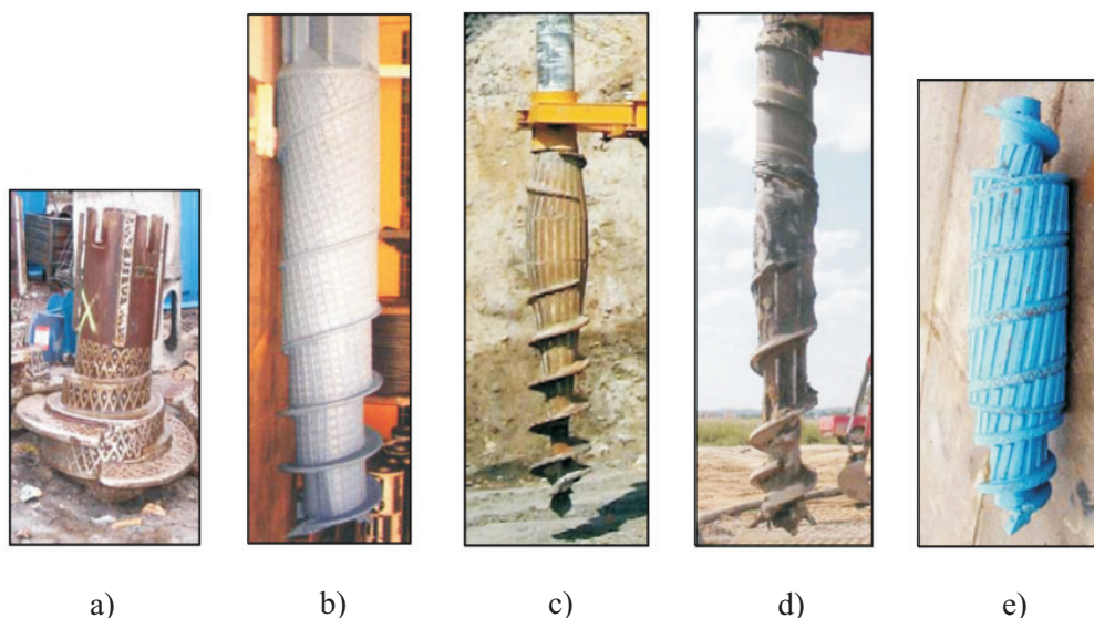
Rys. 1. Przykłady świderów do pali przemieszczeniowych wkręcanych: a) „Atlas”, b) „Omega” – wersja oryginalna [13], c) SDP (FDP) [14], d) CMC [6], e) „Omega” – wersja fińska [3] Fig. 1. Samples of screw displacement pile augers: a) „Atlas”, b) „Omega” – original version [13], c) SDP (FDP) [14], d) CMC [6], e) „Omega” – Finnish version [3]
