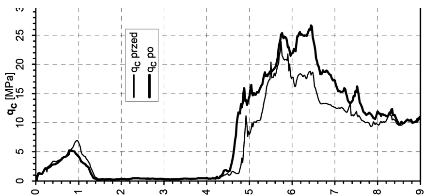
Rys. 13. Rozkłady pionowe siły w kolumnie SDC-b2 otrzymane z pomiarów odkształceń trzonu Fig. 13. Vertical distribution of axial force along SDC-b2 column measured by extensometers
