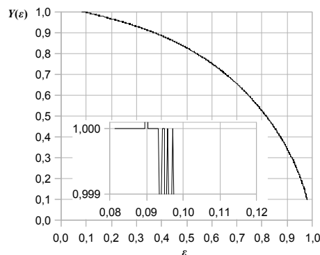
Rys. 5. Funkcja ekspansji Y(\varepsilon) analizowanego elementu pneumatycznego Fig. 5. Expansion function Y(\varepsilon) of the analysed pneumatic circuit
