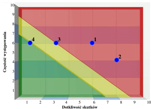
Rys. 2. Matryca ryzyka dla wariantów konstrukcji opisanych w tab. 3
