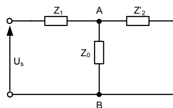
Rys. 3. Schemat zastępczy maszyny indukcyjnej z wirnikiem klatkowym dla stanu ustalonego
