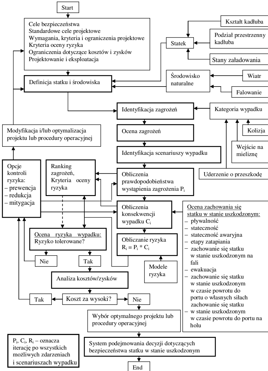
Rys. 1. Struktura metody oceny bezpieczeństwa statków w stanie uszkodzonym, opartej na zachowaniu się statku w stanie uszkodzonym i analizie ryzyka [1]
