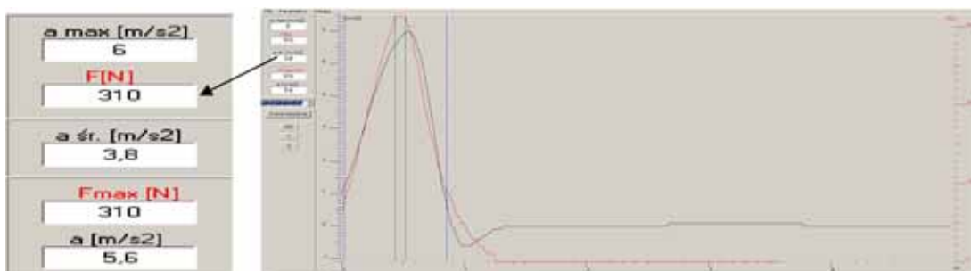
Rys. 4. Wykres opóźnienia hamowania i siły naciski na pedał hamulca. Ciśnienie w ogumieniu kół 2,4 bar
