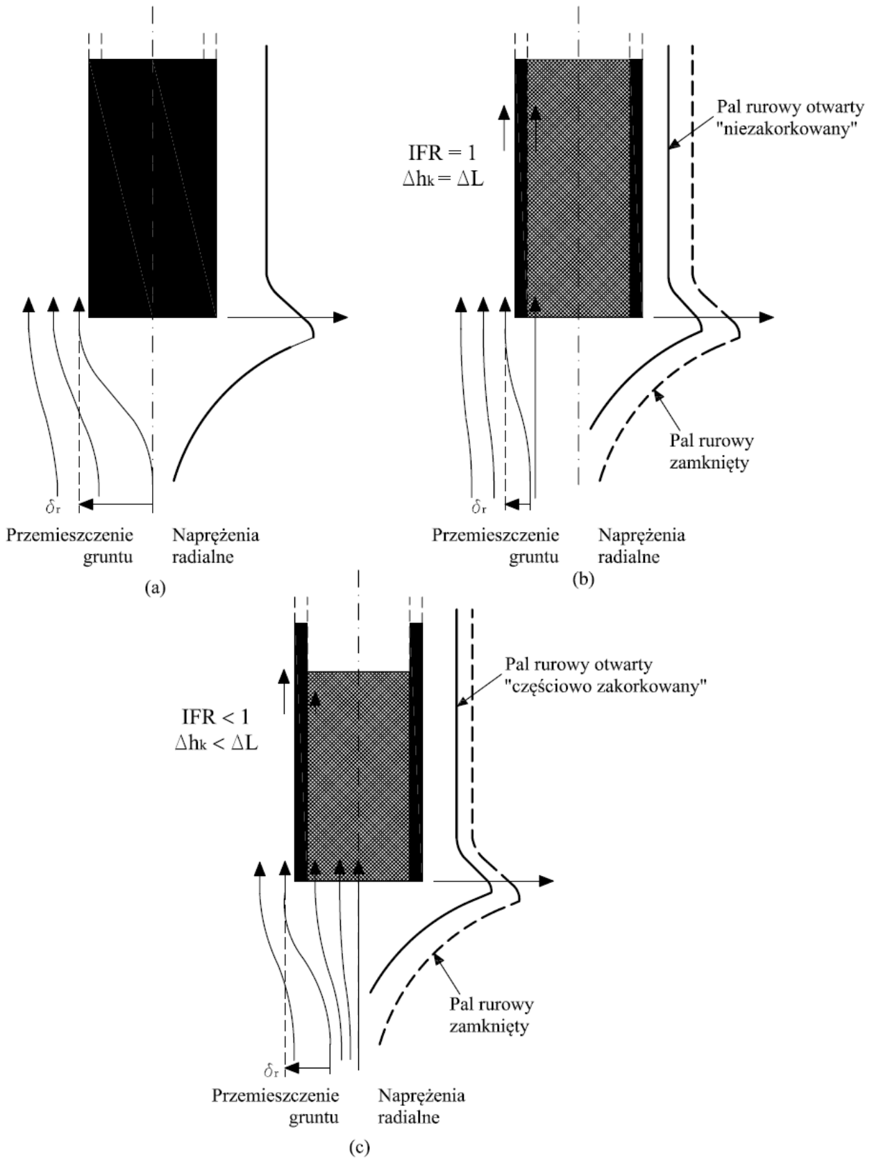
Rys. 2 Proces korkowania pąla ze schematycznie naniesionym kierunkiem przemieszczania się gruntu i naprężeniami radialnymi, (a) pal rurowy zamknięty ( IFR=0 , A_{r,eff} = 1 ), (b) pal rurowy otwarty „niezakorkowany” ( IFR=1 , A_{r,eff} \sim 0,1 ), (c) pal rurowy otwarty „częściowo zakorkowany” ( IFR < 1 , 0,1 < A_{r,eff} < 1 ) [24]
