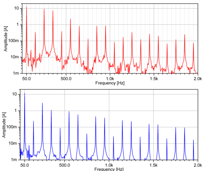
Rys. 5. Porównanie widm składowych harmoniczných prądu wejściowego prostownika 6-pulsowego z obciążeniem pojemnościowym: bez filtracji (wykres górny) oraz z filtracją pasywną (wykres dolny)
