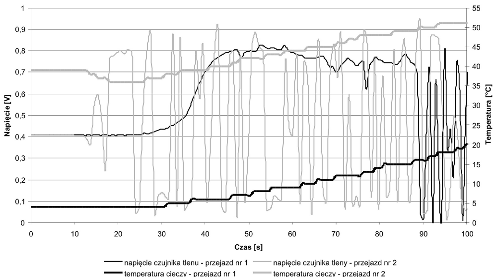
Rys. 8. Napięcie czujnika stężenia tlenu i temperatura cieczy chłodzącej na początku jazd miejskich dla 2 różnych wartości początkowych temperatury cieczy chłodzącej
