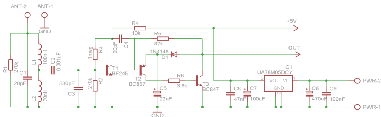
Rys. 7. Schemat wykonanego układu detekcji wyładowań ESD
