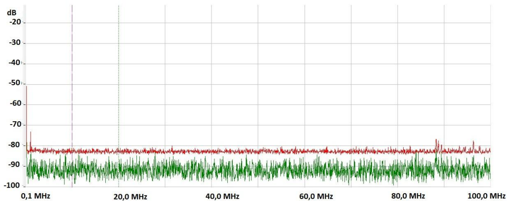
Rys. 4. Zarejestrowana składowa magnetyczna dla pasma 0,1 MHz - 100 MHz przy napięciu wyładowania ESD +1 kV
