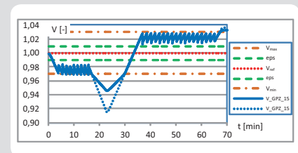
Rys. 11. Zmienność napięcia na szynach stacji GPZ po stronie SN. Przypadek U_{\text{SEE}} = \text{var} oraz \text{tg}\varphi_z = -0,2
