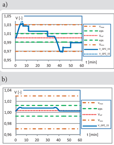
Rys. 13. Zmienność napięcia na szynach stacji GPZ po stronie SN w przypadku P_{gFW} = \text{var} oraz a) \text{tg}(\varphi)_z = -0,2 , b) \text{tg}(\varphi)_z = 0
