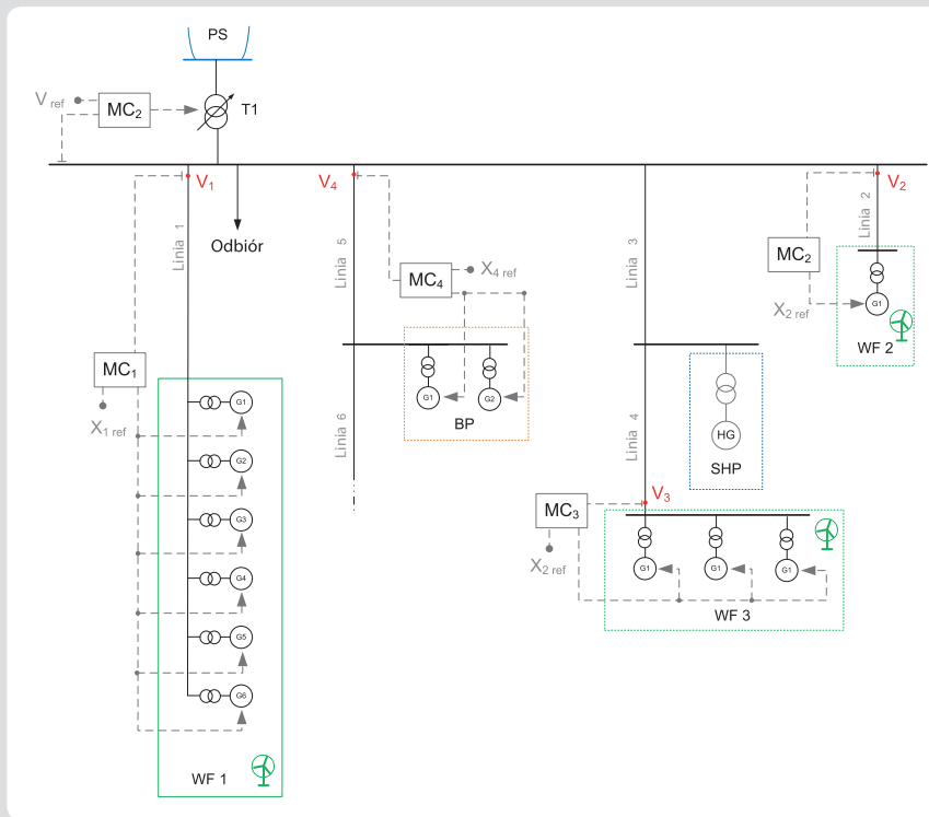
Rys. 3. Uproszczony schemat systemu przyjętego do badań 2
