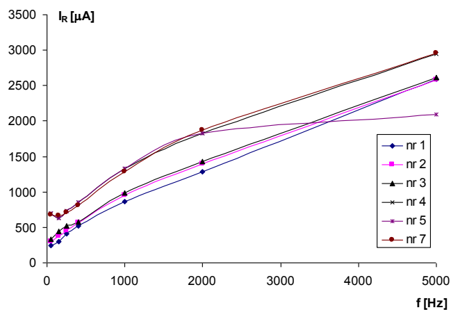
Rys. 8. Wpływ częstotliwości napięcia przemiennego o wartości 325 V na poziom składowej czynnej prądu upływowego
