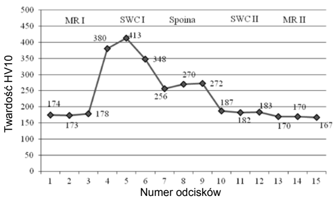
Rys. 23. Rozkład twardości. Próbkę 4BW/a, spawana bez izolacji, linia pomiarowa I, HV10 max = 413
