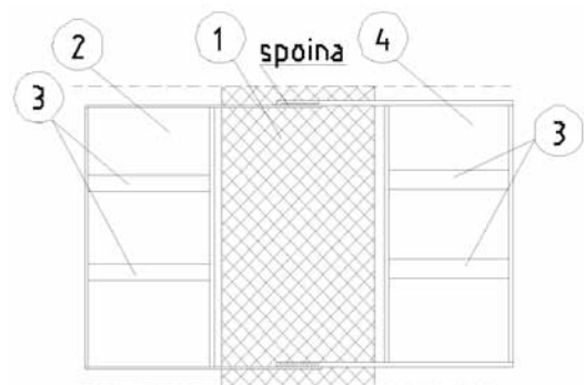
Rys. 4. Widok z góry na skrzynię zamontowaną na stanowisku badawczym: 1 – żelbetonowa kładka; 2 – skrzynia z podklejoną do dna izolacją; 3 – usztywnienia łebkowe; 4 – skrzynia bez izolacji
