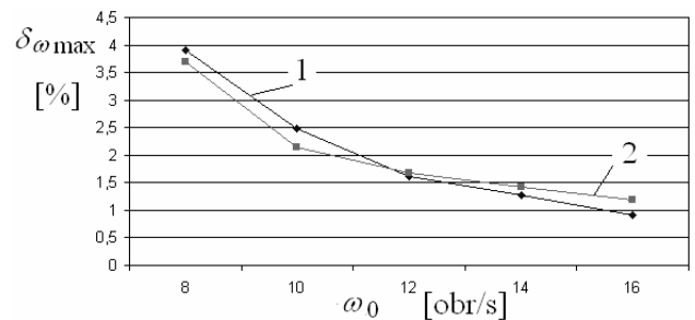
Rys. 7. Maksymalny błąd względny w funkcji \omega_0 dla \omega_m = 2 obr/s, f_p = 50 Hz, \Delta\omega_{zmax} = 0,05 obr/s, C_e = 500 , f_g = 20 MHz; pomiar z: 1 – pojedynczego okresu, 2 – dwóch okresów
