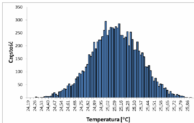
Rys. 3. Histogram dla temperatury 25,1 °C
