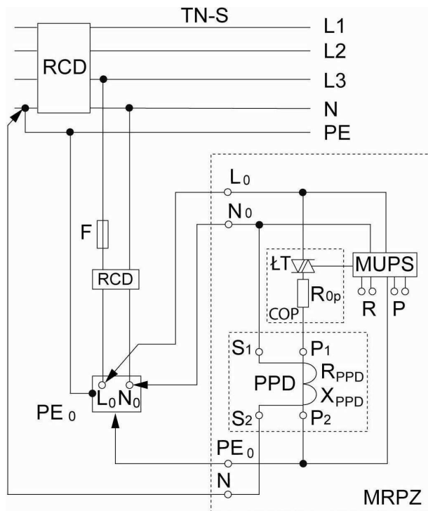
Rys. 5. Schemat blokowy modelu nowego miernika do pomiaru impedancji pętli zwarciowej bez wyzwolenia RCD
