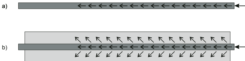
Rys. 3. Fala propagująca w pręcie: a) otoczonym powietrzem; b) osadzonym w betonie
