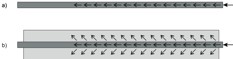
Rys. 3. Fala propagująca w pręcie: a) otoczonego powietrzem; b) osadzonego w betonie
