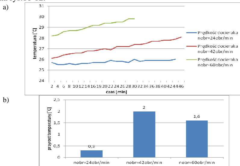
Rys.9. Wyniki badań temperatury rolki regulującej ruch pierścienia prowadzącego: a) w funkcji czasu, b) przyrost temperatury (dla n_{obr} = 24 i 42 \text{ min}^{-1} po 45 min oraz dla n_{obr} = 60 \text{ min}^{-1} – po 30 min)
