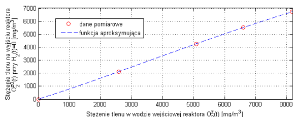
Rys. 6. Zależność stężenia tlenu w wodzie wyjściowej reaktora od stężenia tlenu w strumieniu zasilającym przy dozowaniu wodoru na poziomie H_2(t) = 0 mg/h
