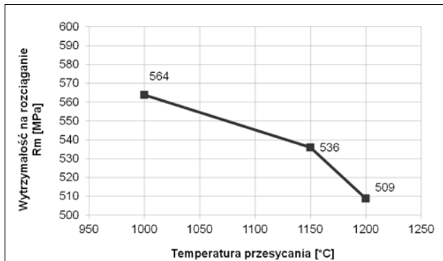
Rys. 7. Zależność wytrzymałości na rozciąganie od temperatury przesycania dla spawanych rurek karbowanych ze stali 316L
