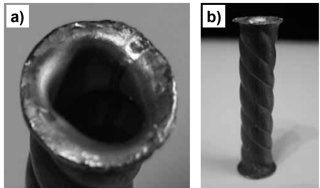
Rys. 10. Próbkę karbowaną po próbie wywijania kołnierza; widok: a) od czoła próbki, b) z boku
