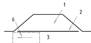
d) Stateczność na wyparcie gruntu spod podstawy nasypu
