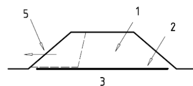
c) Poślizg w nasypie
