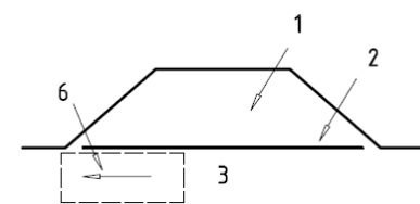
d) Stateczność na wyparcie gruntu spod podstawy nasypu
