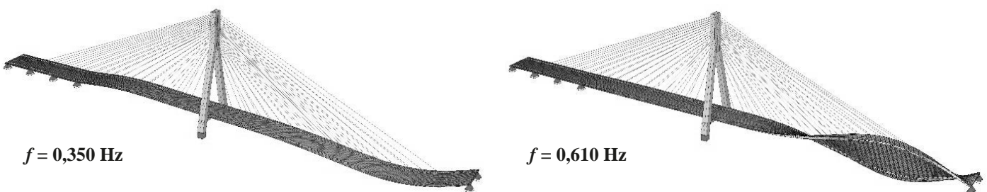
Rys. 12. Pierwsze formy drgań własnych
