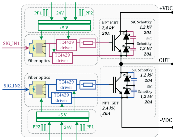
Rys. 2. Schemat opracowanego półmostka IGBT 2,4 kV, 20 A z szybkimi diodami zwrotnymi z węgla krzemu, jako najmniejszego podstawowego energoelektronicznego modułu funkcjonalnego do realizacji strony SN transformatora inteligentnego
