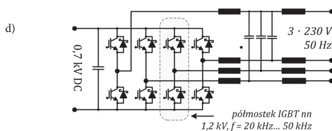
Rys. 1. Inteligentny transformator dystrybucyjny SN/nn: schemat (a), gałęź fazowa AC-DC po stronie SN złożona z połączonych szeregowo mostków tranzystorowych (b), stopień pośredni DC-DC z transformatorem wysokiej częstotliwości dołączany z jednej strony do każdego mostka gałęzi fazowej SN, a z drugiej połączony ze wspólnym przekształtnikiem DC-AC po stronie nn (c), przekształtnik DC-AC po stronie nn (d)
