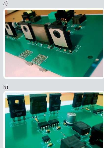
Rys. 3. Widok opracowanego półmostka IGBT 2, 5 kV, 20 A z szybkimi diodami zwrotnymi z węgla oraz zintegrowanymi obwodami sterowania bramkowego (na fotografii zdjęty radiator chłodzący)
