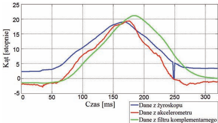
Rys. 15. Działanie filtra komplementarnego Fig. 15. Results of working the complementary filter
