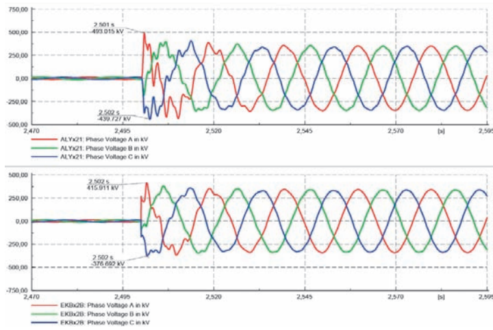
Rys. 6. Napiecia fazowe na końcach toru II linii EKB-ALY
