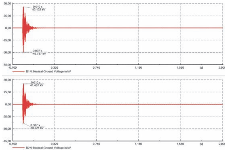
Rys. 5. Napiecia w punkcie gwiazdowym dławików liniowych przyłączonych do szyn stacji Elk Bis
