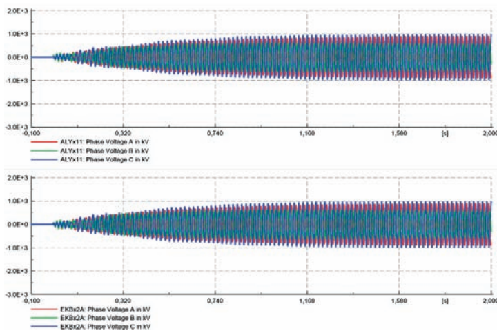
Rys. 7. Napiecia fazowe na końcach wyłączonego toru I linii EKB-ALY
