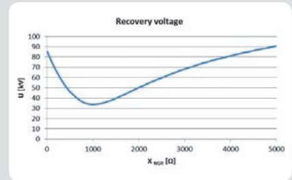
Rys. 9. Napiecia w miejscu zwarcia po jego przemięciu (ang. recovery voltage ). Zwarcie „łukowe” modelowane rezystancją R = 50 \Omega
