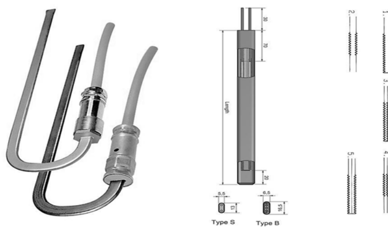
Rys. 4. Grzałka płasko-owalna przeznaczona do pracy w EOR [5]
