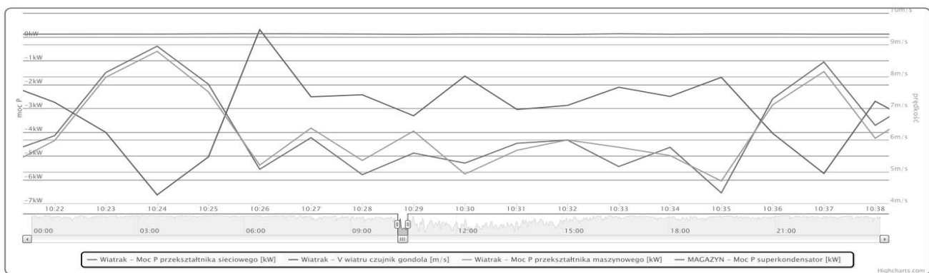
Rys. 8. Przebiegi mocy przetłaczalnika maszynowego, sieciowego i prędkości wiatru zarejestrowane przez system ECV-2.0
