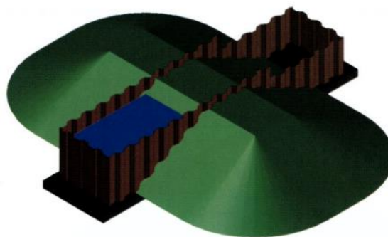
Rys. 2. Schemat stanowiska modelowego wału przeciwpowodziowego 11
