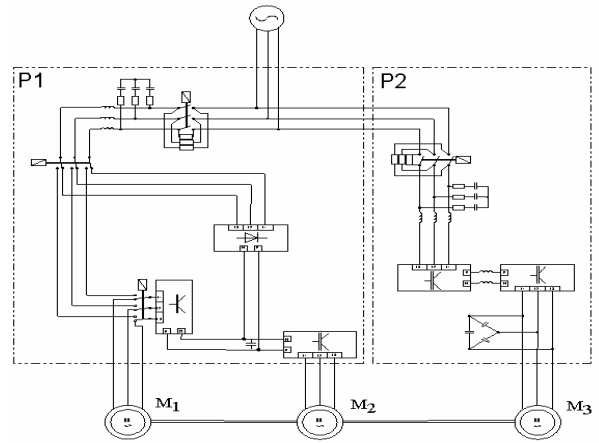
Rys. 6. Schemat stanowiska laboratoryjnego
