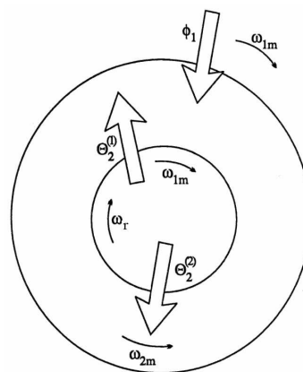
Rys. 1. Składowe przepływy w asymetrycznym wirniku [1]
