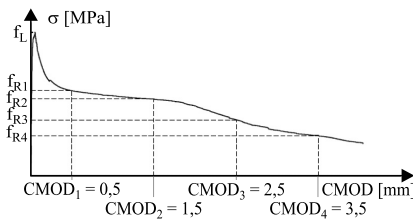
Rys. 3. Schematyczny wykres naprężenie rozciągające – rozwarście krawędzi szczeliny CMOD przy badaniu wytrzymałości resztkowej na zginanie wg PN-EN 14651 [7] Fig. 3. Schematic diagram of tensile stress – crack mouth opening displacement (CMOD) according to EN 14651 [7]
