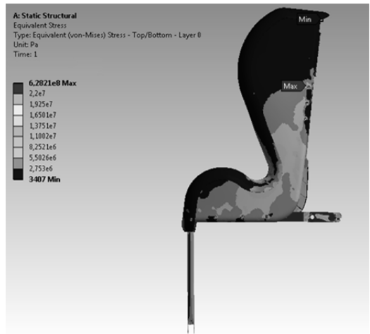
Rys. 11. Wyniki analizy: naprężenia zredukowane, widok z boku [1]
