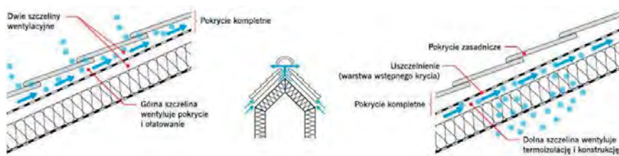
Rys. 14. Zasada działania wentylacji: w dachu z dwiema szczelinami (www.infoarchitekta.pl)
