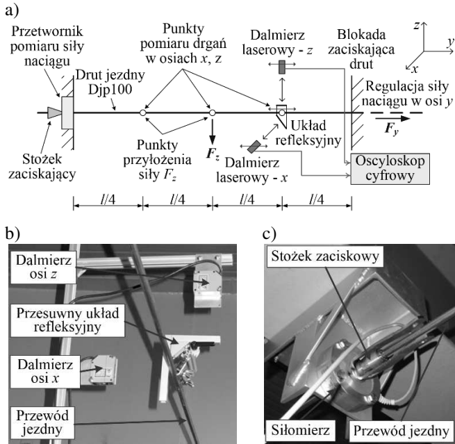
Rys. 1. Laboracyjne stanowisko pomiarowe: a) szkic struktury; b) zespół dalmierzy laserowych i płytek refleksyjnych na przewodzie; c) przetwornik do pomiaru siły naciągu przewodu
