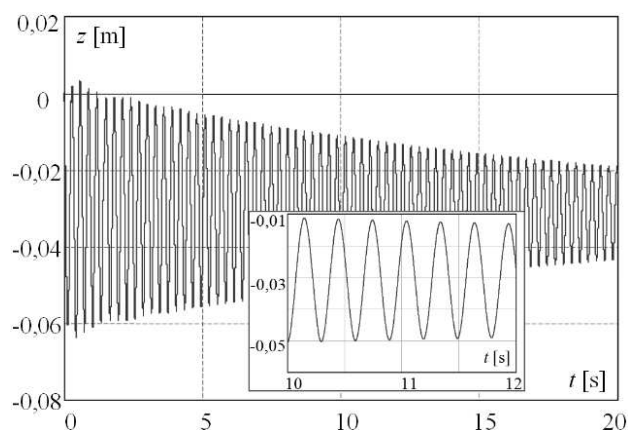
Rys. 9. Wynik symulacji drgań odcinka przewodu jezdnego
