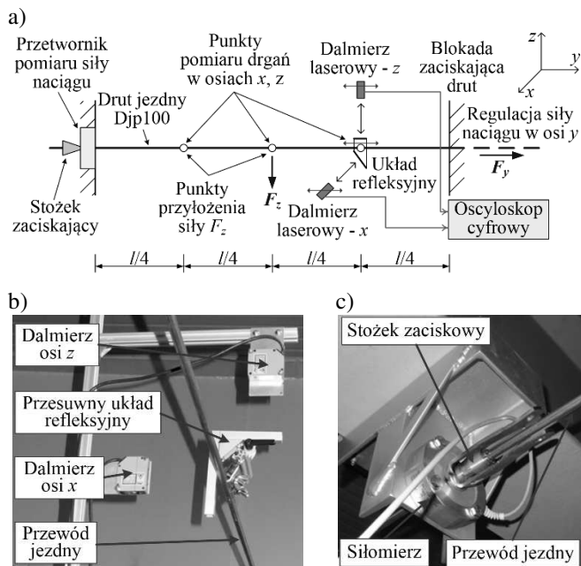
Rys. 1. Laboracyjne stanowisko pomiarowe: a) szkic struktury; b) zespół dalmierzy laserowych i płytek refleksyjnych na przewodzie; c) przetwornik do pomiaru siły naciągu przewodu
