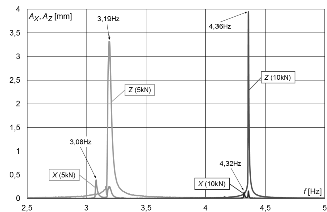
Rys. 3. Charakterystyka widmowa drgań przewodu Dj100 dla warunków jak na rys. 2
