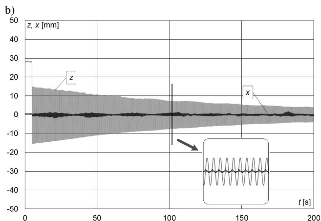
Rys. 2. Drgania przewodu jezdnego Djp 100 w osi z (pionowej) i w osi x (poziomej), po odcięciu skokową siłą pionową 100 N w 1/2 rozpiętości odcinka przewodu o długości 12 m, przy rejestracji drgań w 1/2 odcinka przy naciągu: a) 5 kN; b) 10 kN
