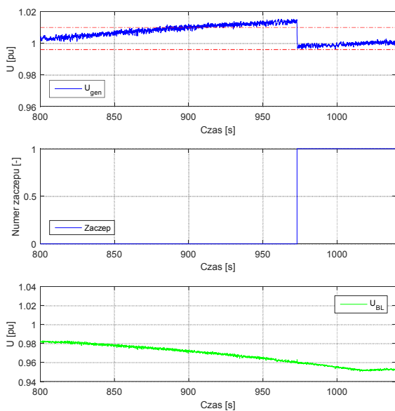
Rys.12. Przebiegi napięć na zaciskach bloku i generatora oraz numeru zaczeputu przy liniowej zmianie mocy biernej odbiornika LOAD1– wariant „B”
