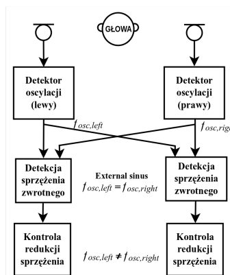
Rys. 9. Redukcja sprzężenia zwrotnego przy użyciu łącza danych pomiędzy dwoma aparatami słuchowymi
