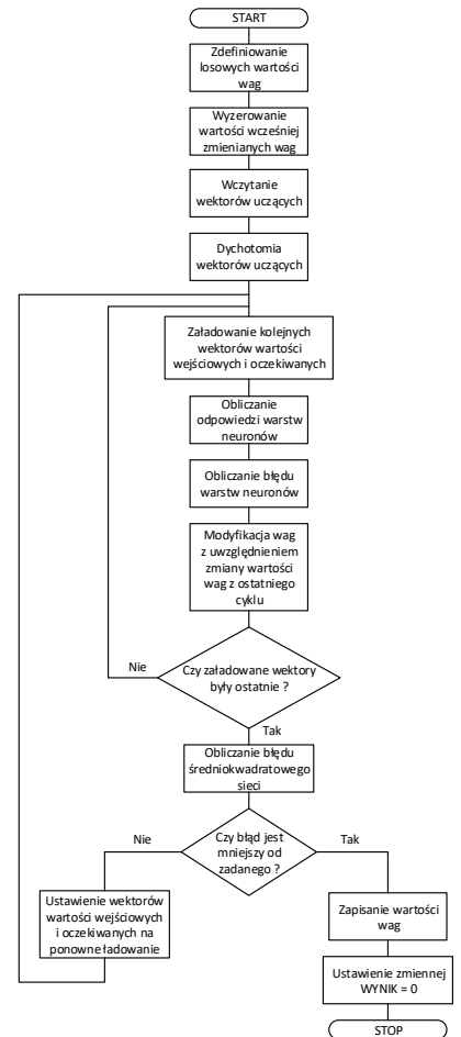
Rys. 6. Algorytm uczenia
