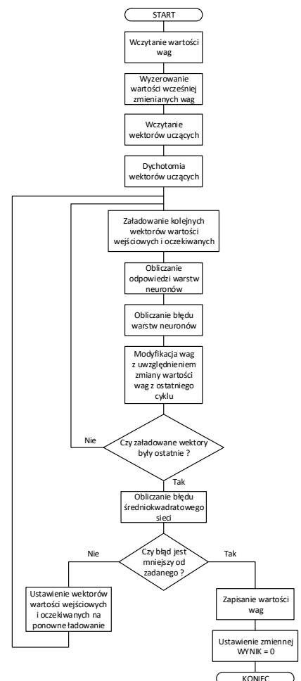
Rys. 7. Algorytm douczania
