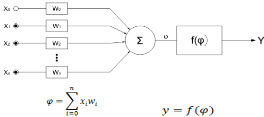
Rys. 1. Schemat neuronu
