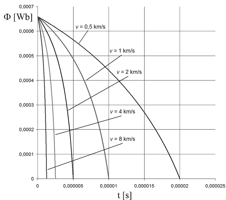
Rys. 7. Przebieg strumienia magnetycznego w układzie dla różnych wartości prędkości odkształcenia dla a = 0,3\text{m} i D/d = 3
